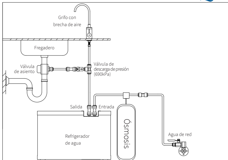
Figura 2. Ilustración de la instalación
