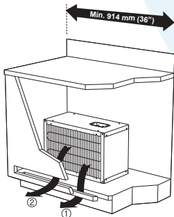
Figura 1. Ventilación adecuada para la instalación
